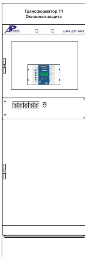
Шкаф основных защит двухобмоточного трансформатора ШЭРА-ДЗТ-1002БПВА.656457.426, БПВА.650645.001 ТУ
